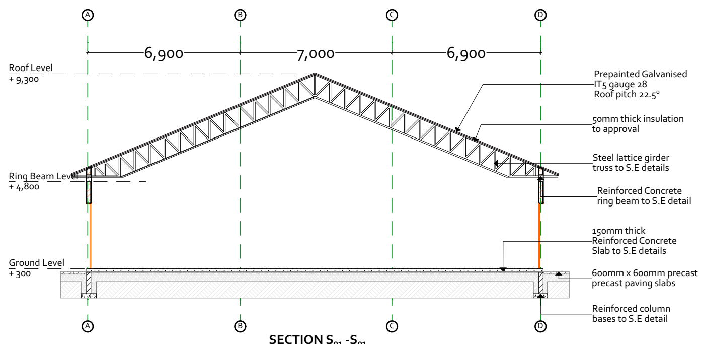
SECTION S 01 -S 01
